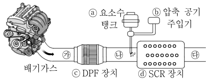
<디젤 엔진의 배기가스 저감 장치>
